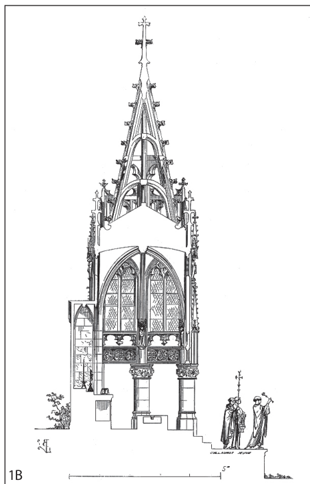
Figur 1. La Recevresse d'Avioth (départ. Meuse, Frankrig). A. Plan. B. Snit. C. Perspektivtegning (Fra Viollet-le-Duc 1875).
