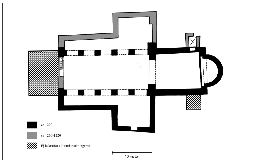
Fig. 4. Edsleskogs medeltida kyrka. Planritning med kyrkans två tidigaste faser under 1200-talet. Bild: Lödöse museum
