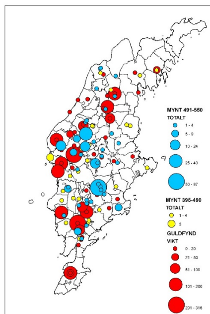
Fig. 9. Total mängd guldfynd på Gotland från folkvandringstid.
