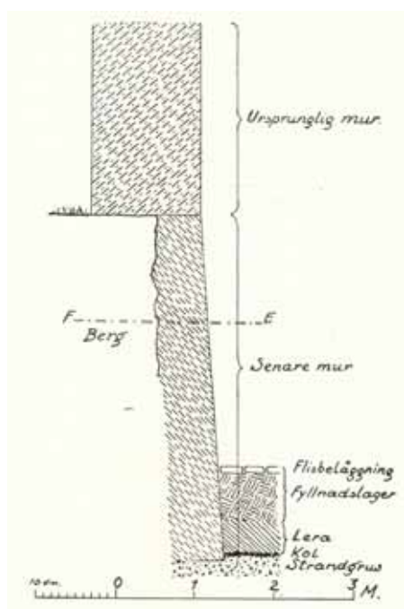
Fig 20. Murprofil. Från undersökning 1925 (Efter Eckhoff & Janse 1936).
