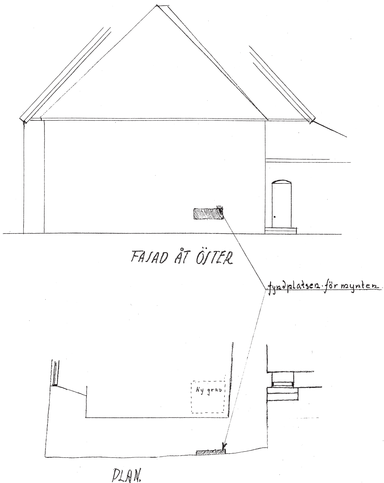
Fig.4, Fasad- och planritning över korets östra del, visande fyndplatsen för de mynt som hittades i kormuren under 1927-28 års restaurering (ritning i ATA, 1927, Dnr 2079).
